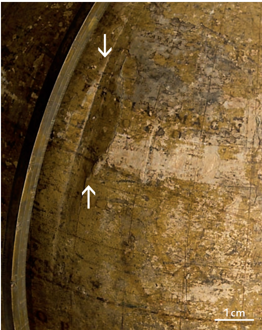
Abb. 11 Nordhalbkugel des Erdglobus (Ausschnitt im Streifenlicht von rechts): konkave Deformation der Globuskugel.
