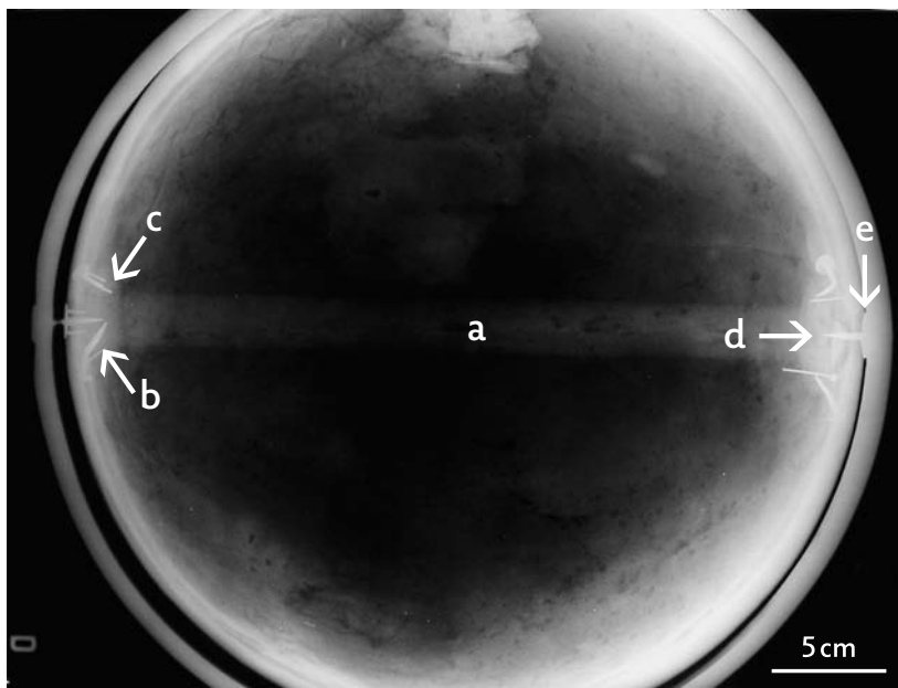
Abb. 6: Erdglobuskugel (Röntgenaufnahme): zentrale Achse (a), mit Nägeln (b) an einem verdickten Teil der Kugelschale (c) befestigt; Nord- und Südpol jeweils mit Achsstift (d), der außen mit einem Metallplättchen (e) verlötet ist.
