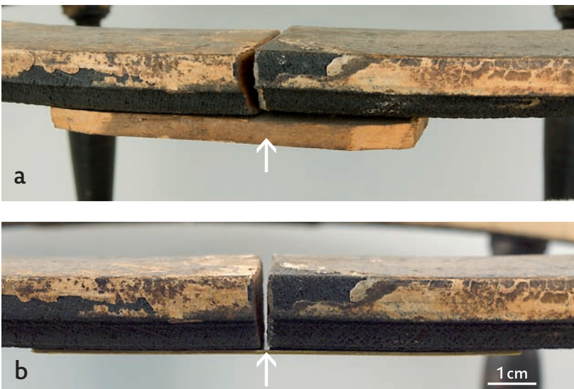
Abb. 16a+b Erdgloбус, Seitenansicht der Horizontringbasis vor und nach der Restaurierung. Das provisorische Holzstück (a) wurde durch eine auf die Horizontringbasis individuell angepasste Metallbrücke (b) ersetzt.
