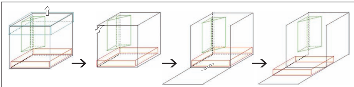
Abb. 18 Schematische Darstellung der Verpackung. Es handelt sich um eine zweiteilige Stülpdeckelbox (blau+grau) mit aufklappbarer Vorderseite. Innen ist sie mit einer Art Schublade (rot) aus Karton ausgestattet, die mit einem Innenbett aus Schaumstoff (orange) gefüllt ist. Hierin befinden sich 4 Ausschnitte für die Füße des Globusstuhls. In den Ecken der Box sind Elemente aus flexiblen, leicht federndem Karton (grün) montiert, die in Berührung mit der Horzontringbasis kommen und den Globus so stabilisieren.
