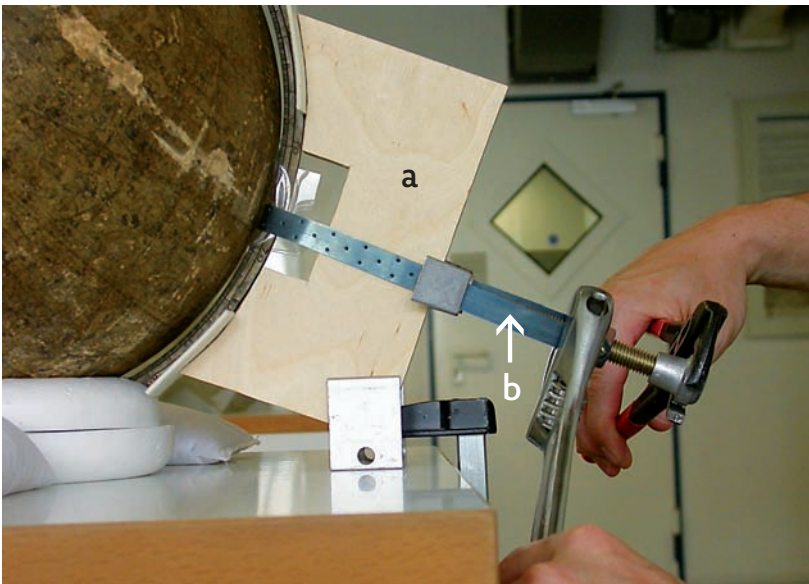
Abb. 14 Vorrichtung zur Minimalisierung der Deformation im Meridianring. Die Holzschablone (a) ermöglicht den Aufbau lokaler Spannung am Meridianring, welche durch einen sogenannten Ölfilter-Löseschlüsselstahl (b) ausgeübt wurde.
