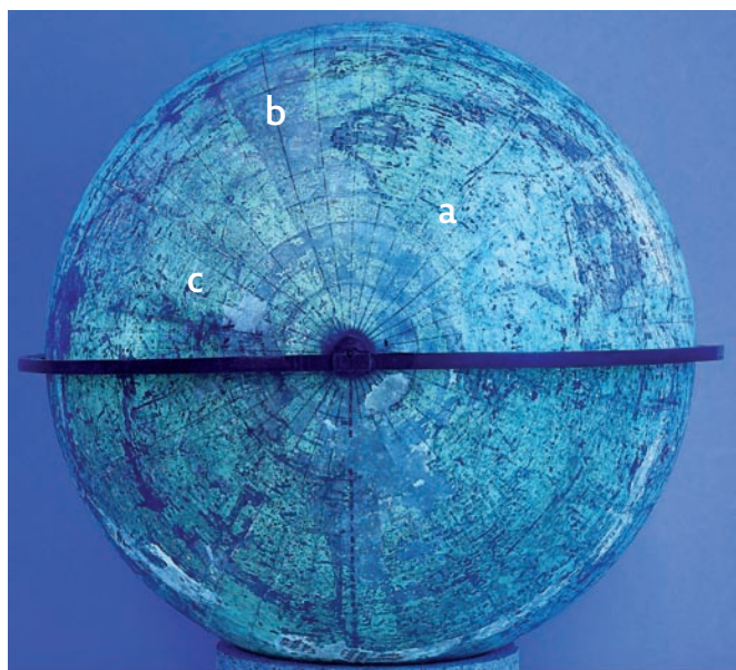
Erdglobus, UV-Aufnahme: vergilbter Firnis (a), Fehlstellen im Firnis mit starker, dunkelfarbiger Anlagerung von Verschmutzungen (b), Eisengallustinte mit Hofbildung (c).
