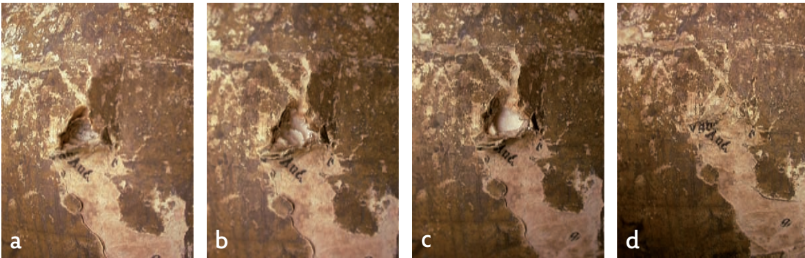
Abb. 13a–d Erdglobus, Detailaufnahmen während der Restaurierung. Hohlräume im Kugelkorpus werden schrittweise mit Japanpapierfasern und wenig Weizenstärkekleister gefüllt und lose Segmentpapiere konsolidiert.
